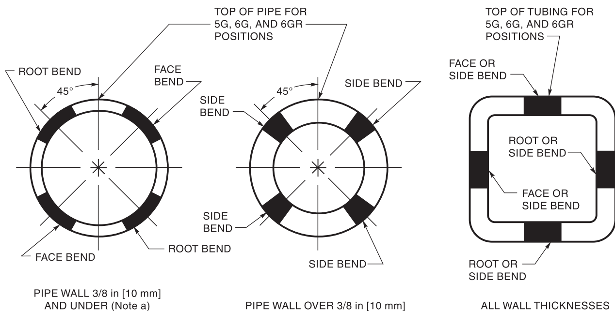
SPECIMENS FOR 5G, 6G, AND 6GR POSITIONS
